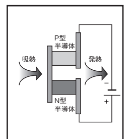
ペルチェ素子の原理
